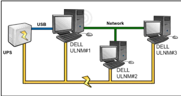
그림 45. 전원 흐름도
