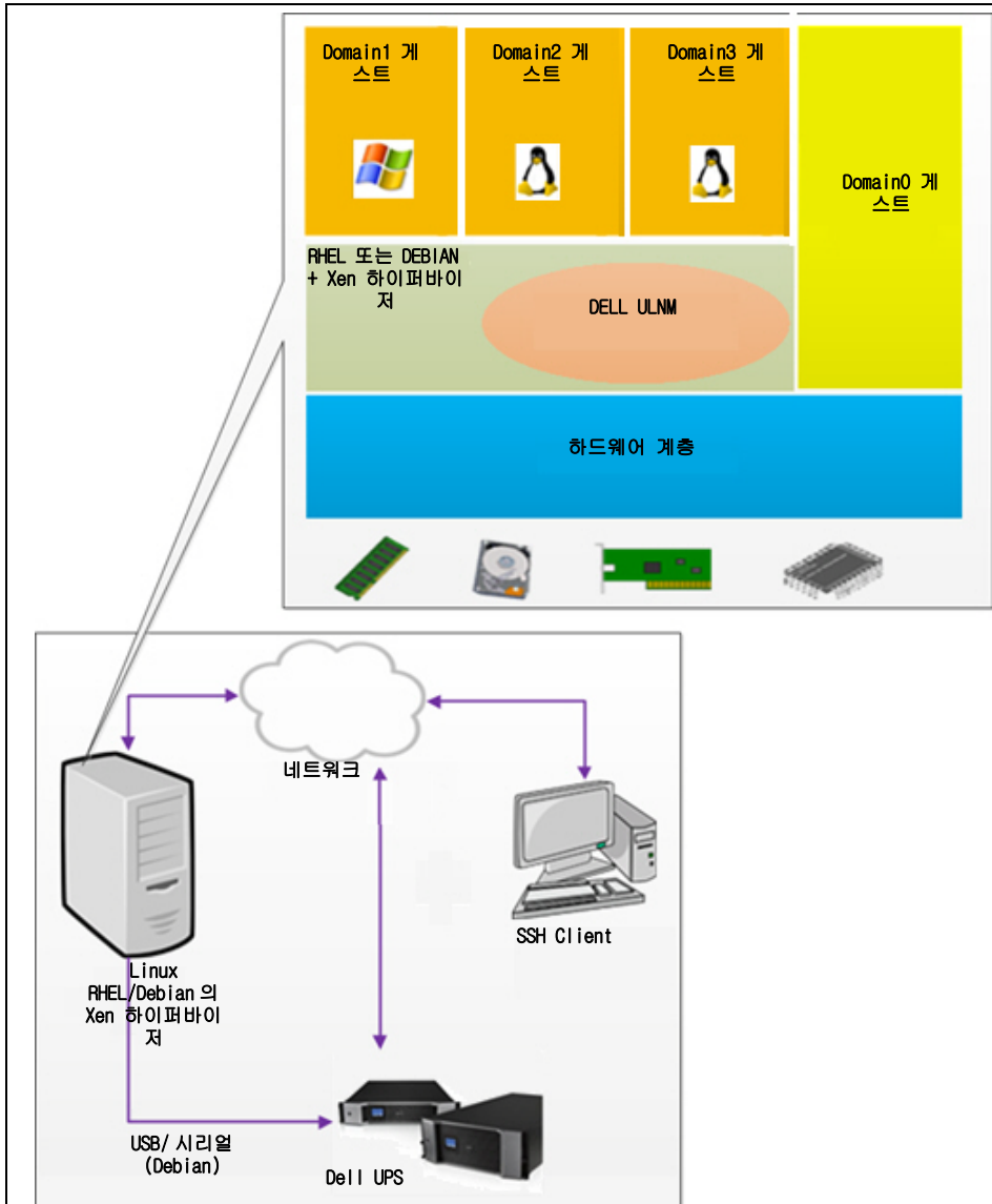
그림 99. Dell ULNM RHEL 5 및 Debian 5.0 아키텍처에 대한 구성
