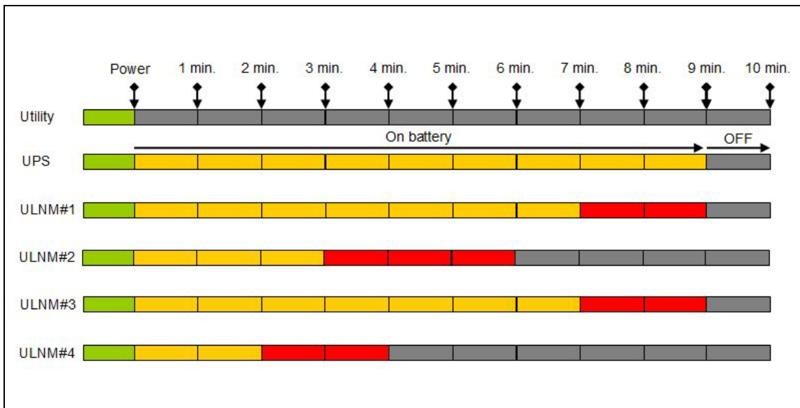
그림 27. 종료 제어기 다이어그램
