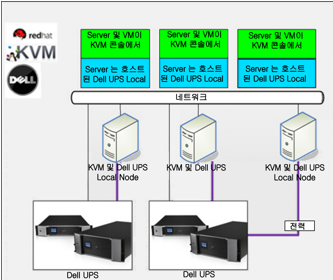
그림 100. Red Hat KVM 또는 오픈소스 KVM 용 Dell ULNM 솔루션
