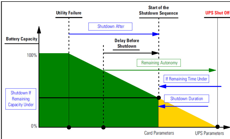
그림 19. 종료 시퀀스
