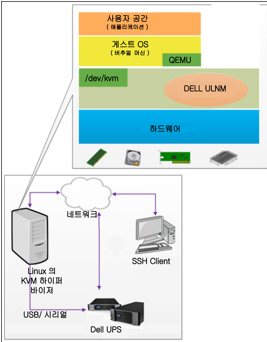
그림 101. Dell ULNM RHEL 6 및 Debian 5.0 아키텍처의 KVM에 대한 구성
